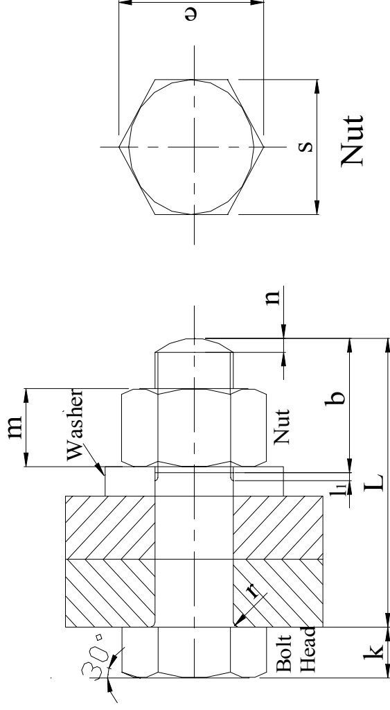
Bolt
