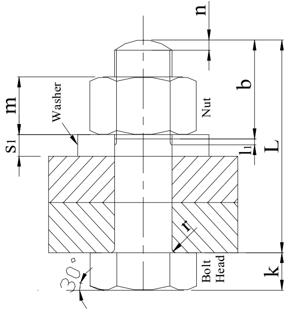
Bolt
